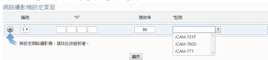
图 6-49: iCAM 网络摄影机型号设定
