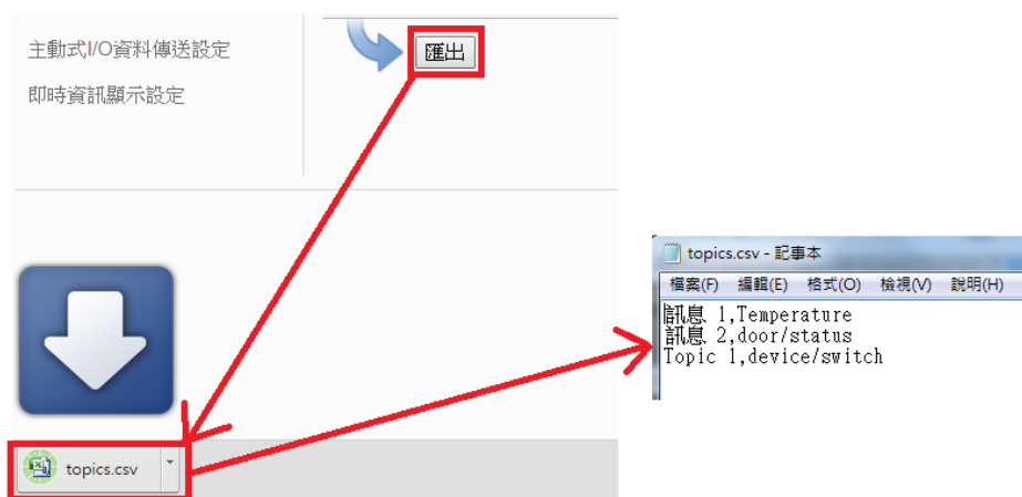
图 8-14: MQTT Topic 汇出
