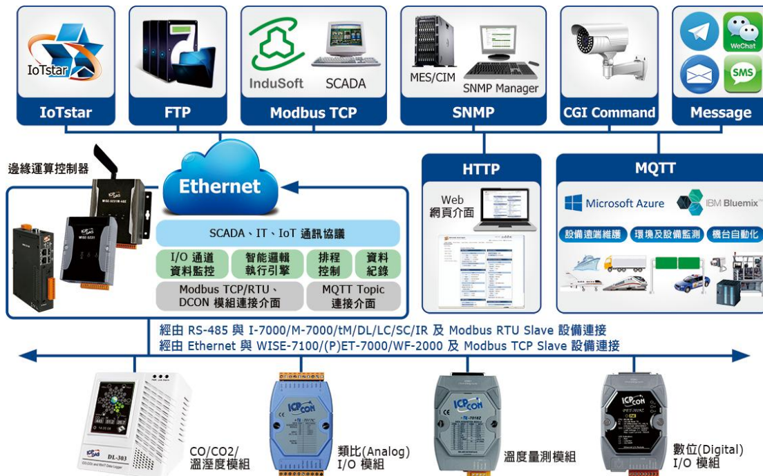
圖 1-1 : WISE-523x/WISE-224x 系統架構圖
